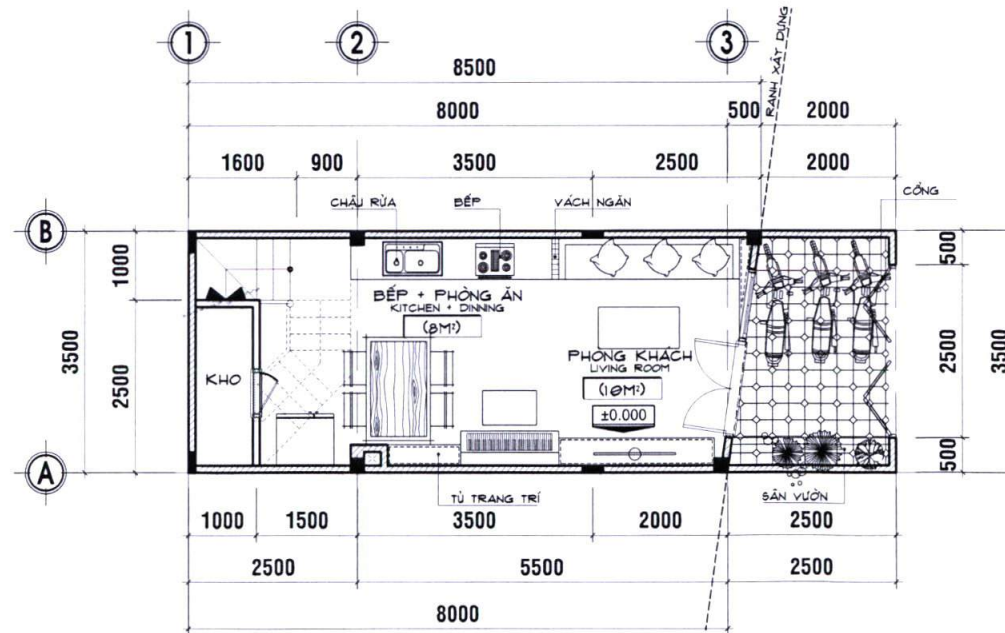
MẶT BẰNG TẦNG 1_TL: 1/100 1ST FLOOR
