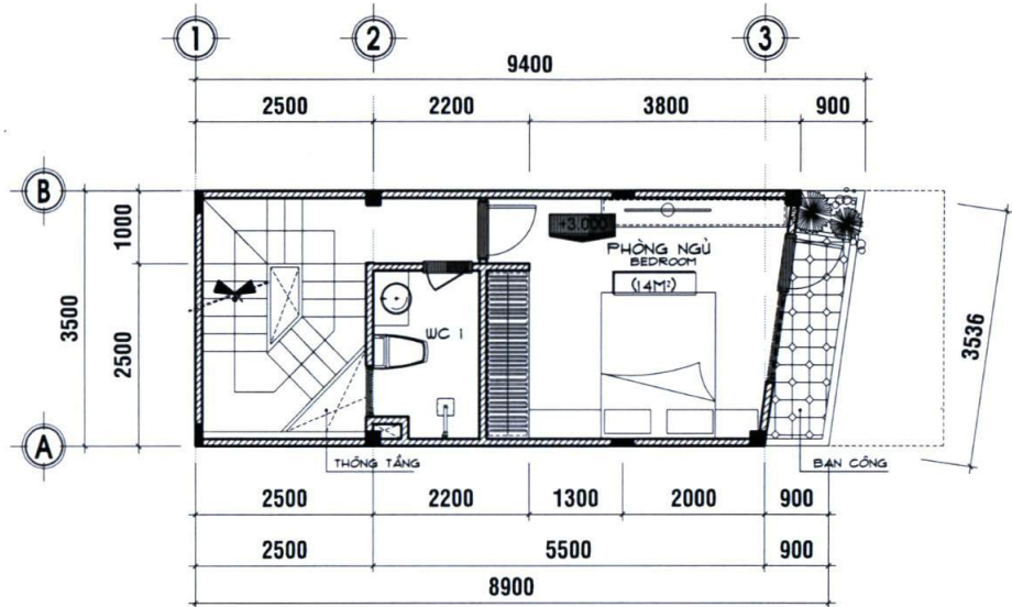
⊕ MẶT BẰNG TẦNG 2_TL: 1/100 2ST FLOOR
