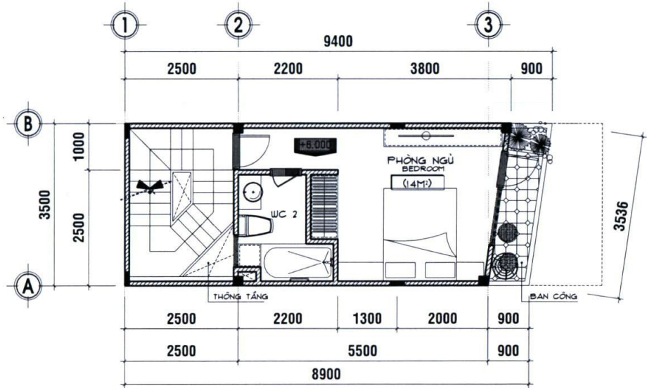
⊕ MẶT BẰNG TẦNG 3_TL: 1/100 3ST FLOOR
